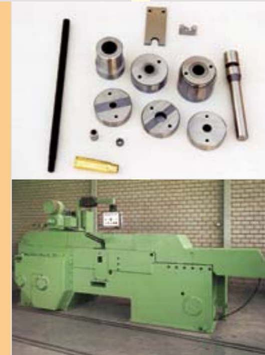
Orta kalibre pres Middle calibre press
